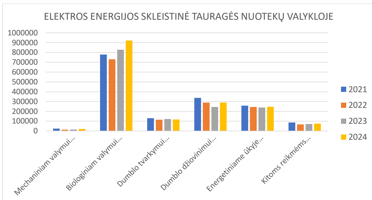
9 pav. Elektros energijos skleistinė Tauragės nuotekų valykloje 2021 – 2024 m.
