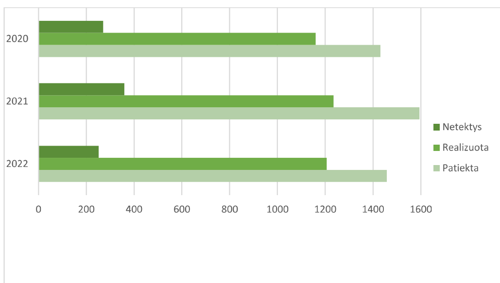
2 pav. UAB „Tauragės vandenys“ vandens tiekimas, realizacija ir netektys 2022m., tūkst. m 3
