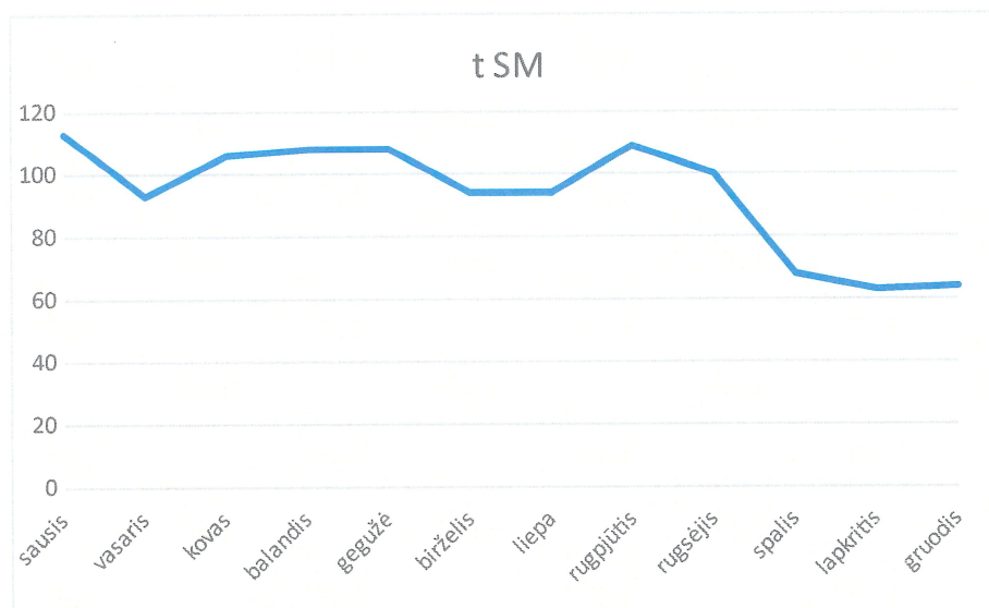
Paveikslas 3. Bendras dumblo kiekis, t SM
